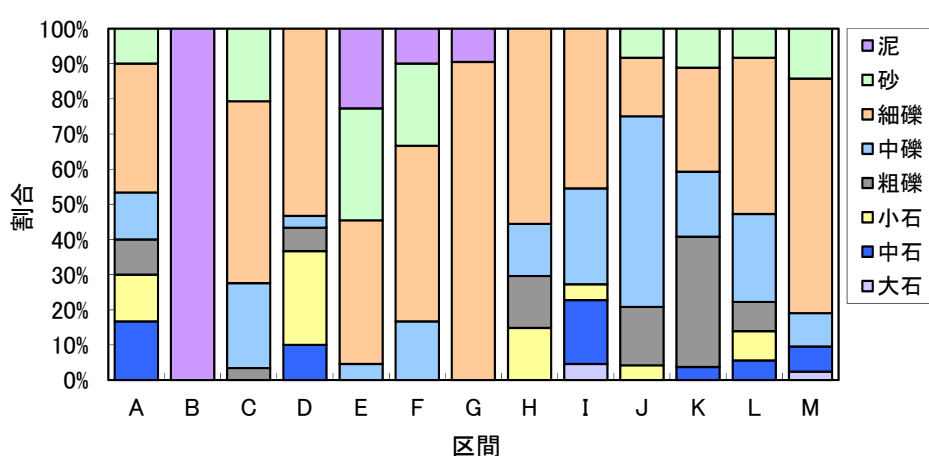
図 3. 10 対象区域内における河床材料の構成割合（各区間の位置は図 3. 11 参照）
