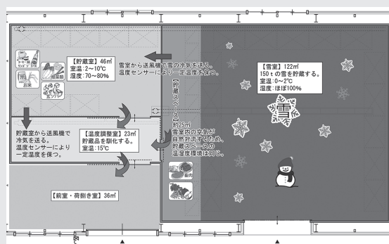
▲「雪室スノーパル」の内面図
